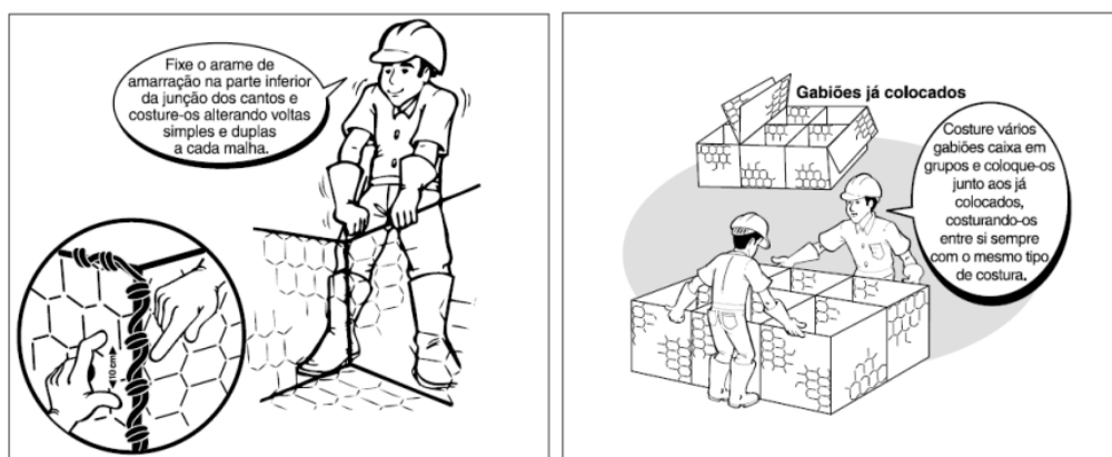
Figura 3: Costura das arestas com o arame de amarração Figura 4: Posicionamento dos gabiões antes do enchimento
